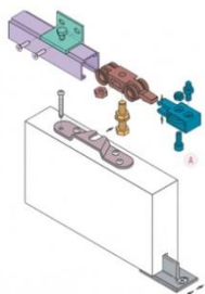
Tolóajtó vasalat szerkezeti felépítése és alkatrészei
