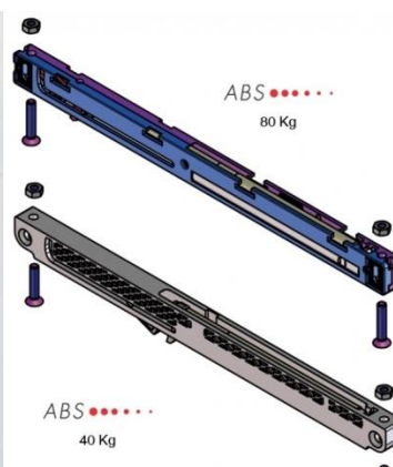
Tolóajtókhoz rendelhető ABS fékezőrendszer
